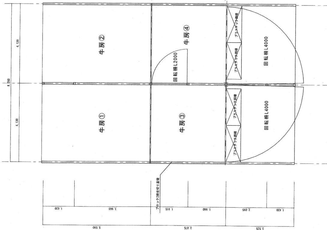
平面図
